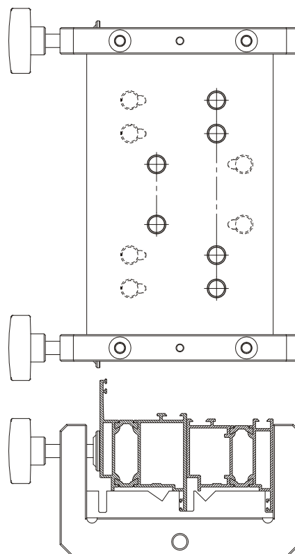
Dima di foratura per cerniere art. 1143.35 per aperture interne. Drilling jig for hinges art. 1143.35 for internal openings. Gabarit de perçage pour la paumelle art. 1143.35 (ouvertures intérieures). Plantilla de taladro para la bisagra art. 1143.35 (aberturas hacia el interior). Bohrschablone für Bänder Art. 1143.35 für Öffnung nach einwärts. Шаблон для сверления к петлям арт. 1143.35 для внутреннего открывания.
