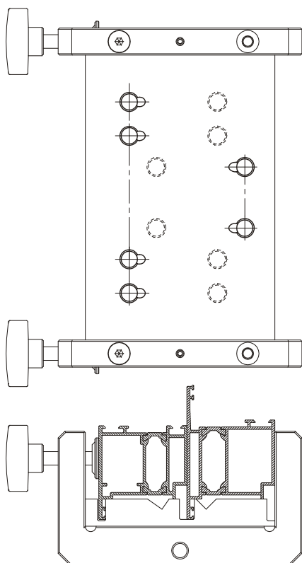
Dima di foratura per cerniere art. 1143.36 per aperture esterne. Drilling jig for hinges art. 1143.36 for external openings. Gabarit de perçage pour la paumelle art. 1143.36 (ouvertures extérieures). Plantilla de taladro para la bisagra art. 1143.36 (aberturas hacia el exterior). Bohrschablone für Bänder Art. 1143.36 für Öffnung nach auswärts. Шаблон для сверления к петлям арт. 1143.36 для наружного открывания.
